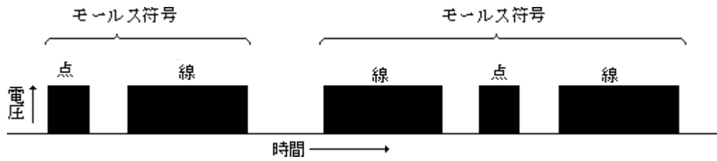
別図第十七号 標識信号の構成(第45条の12の10関係)
