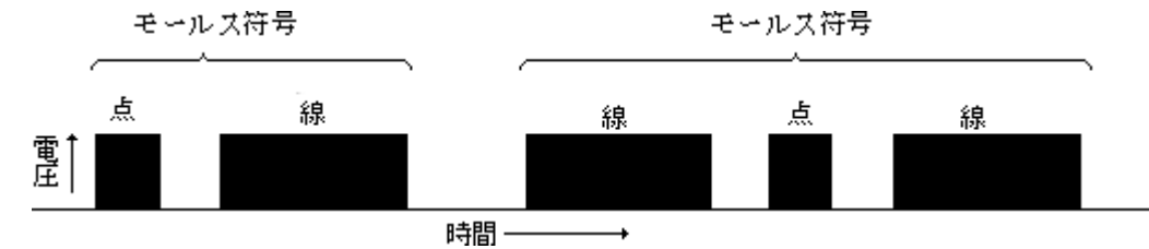
別図第十七号 標識信号の構成(第45条の12の10関係)
