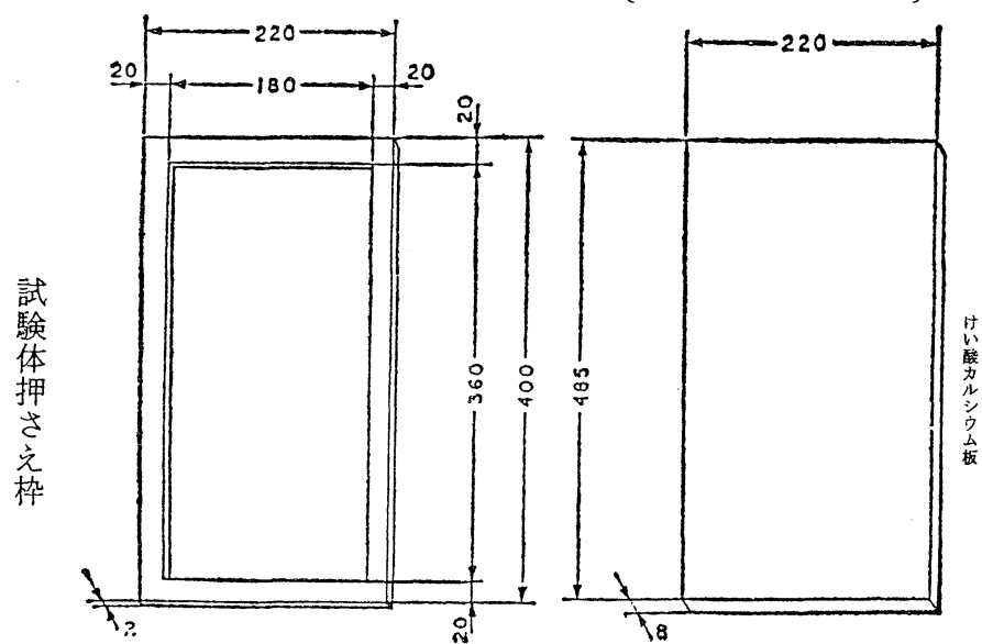
別図第2の3 試験体押さえ枠及びけい酸カルシウム板(第4条の3関係) (単位 ミリメートル)
