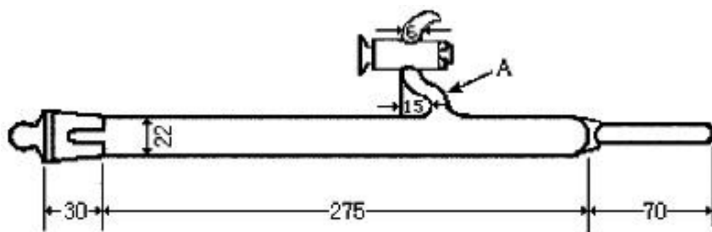
リョーリツヒ管 (単位mm)
